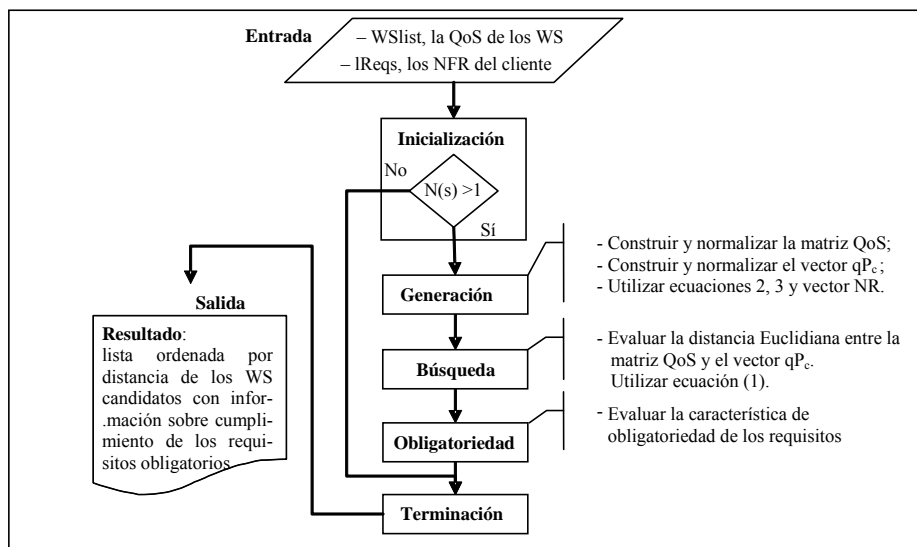
Figura 5. Algoritmo del módulo de selección
