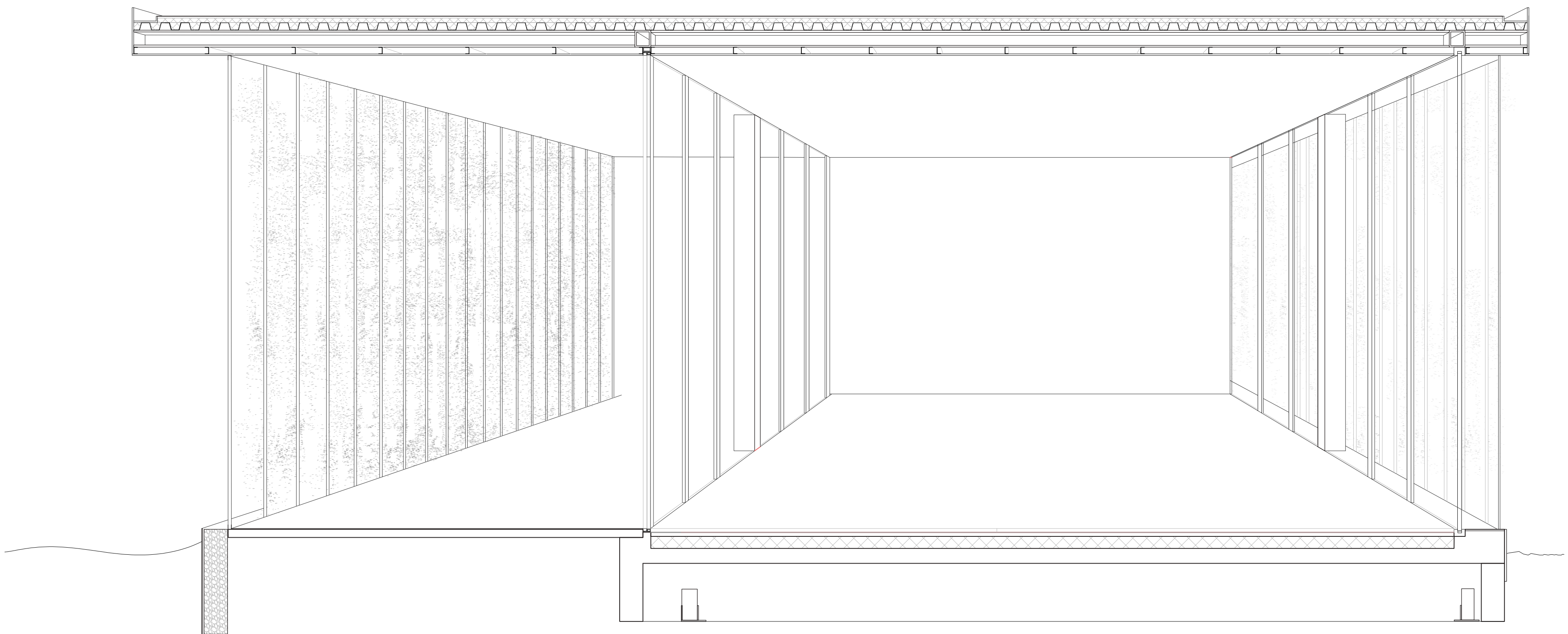
SECCION CONSTRUCTIVA DEL TALLER DE TRABAJO PARA LOS RESIDENTES E 1:20
