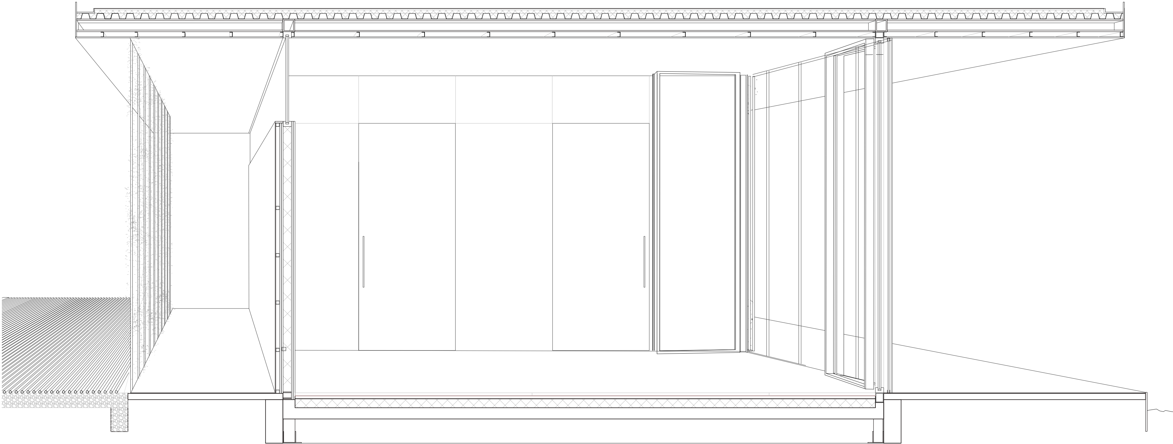
SECCIÓN CONSTRUCTIVA HABITACIÓ RESIDENCIA E 1:20
