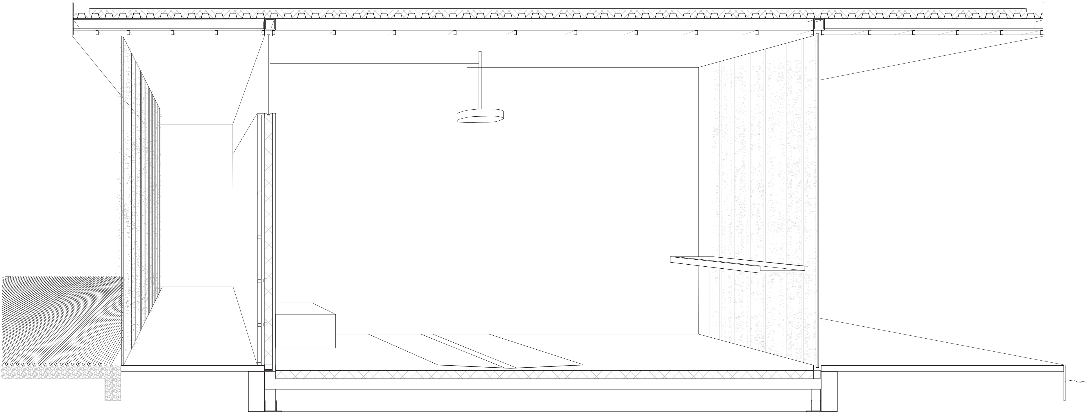
SECCIÓN CONSTRUCTIVA LAVABO RESIDENCIA E 1:20
