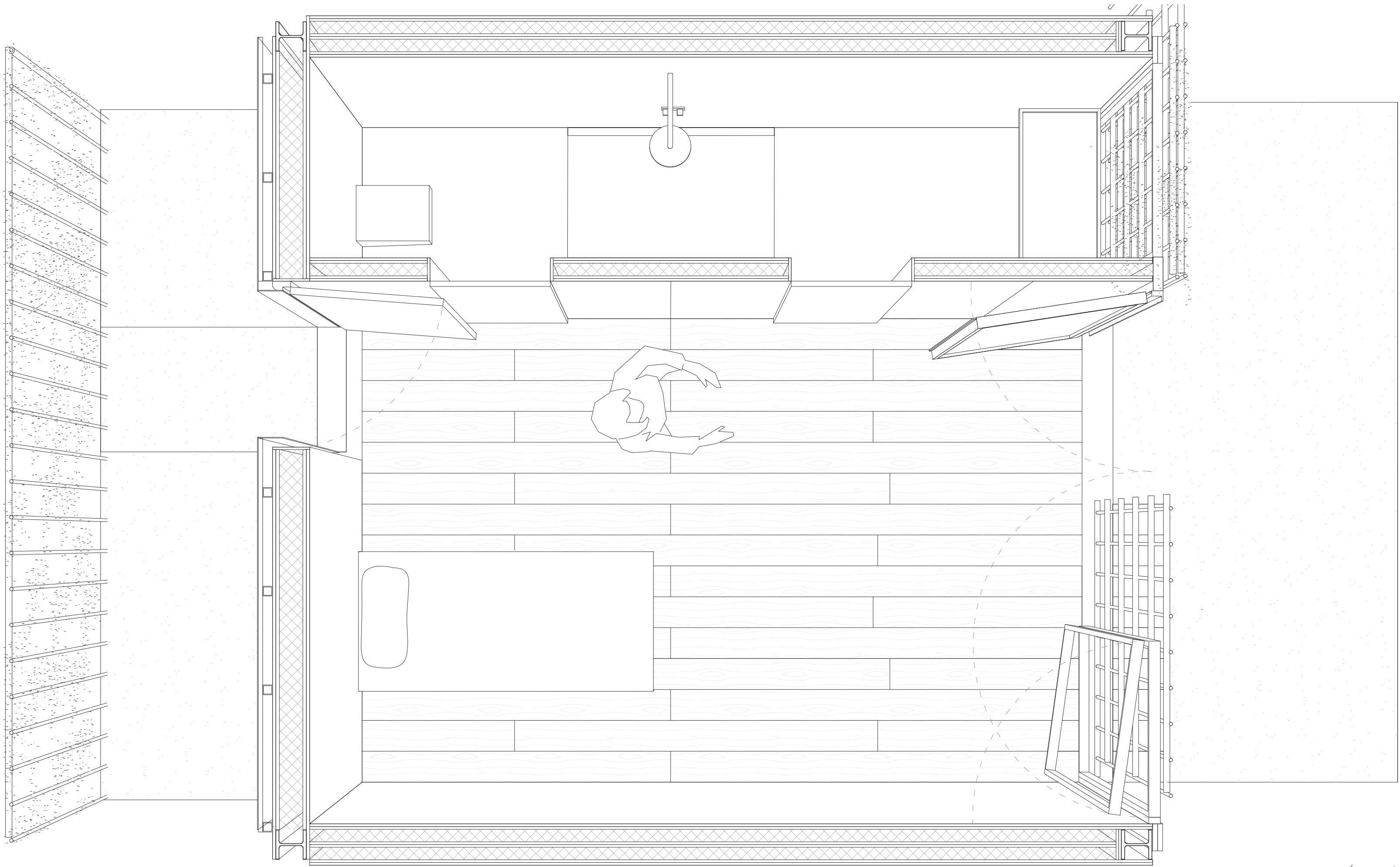
PLANTA DE UN MÓDULO DE LA RESIDENCIA E 1:20
