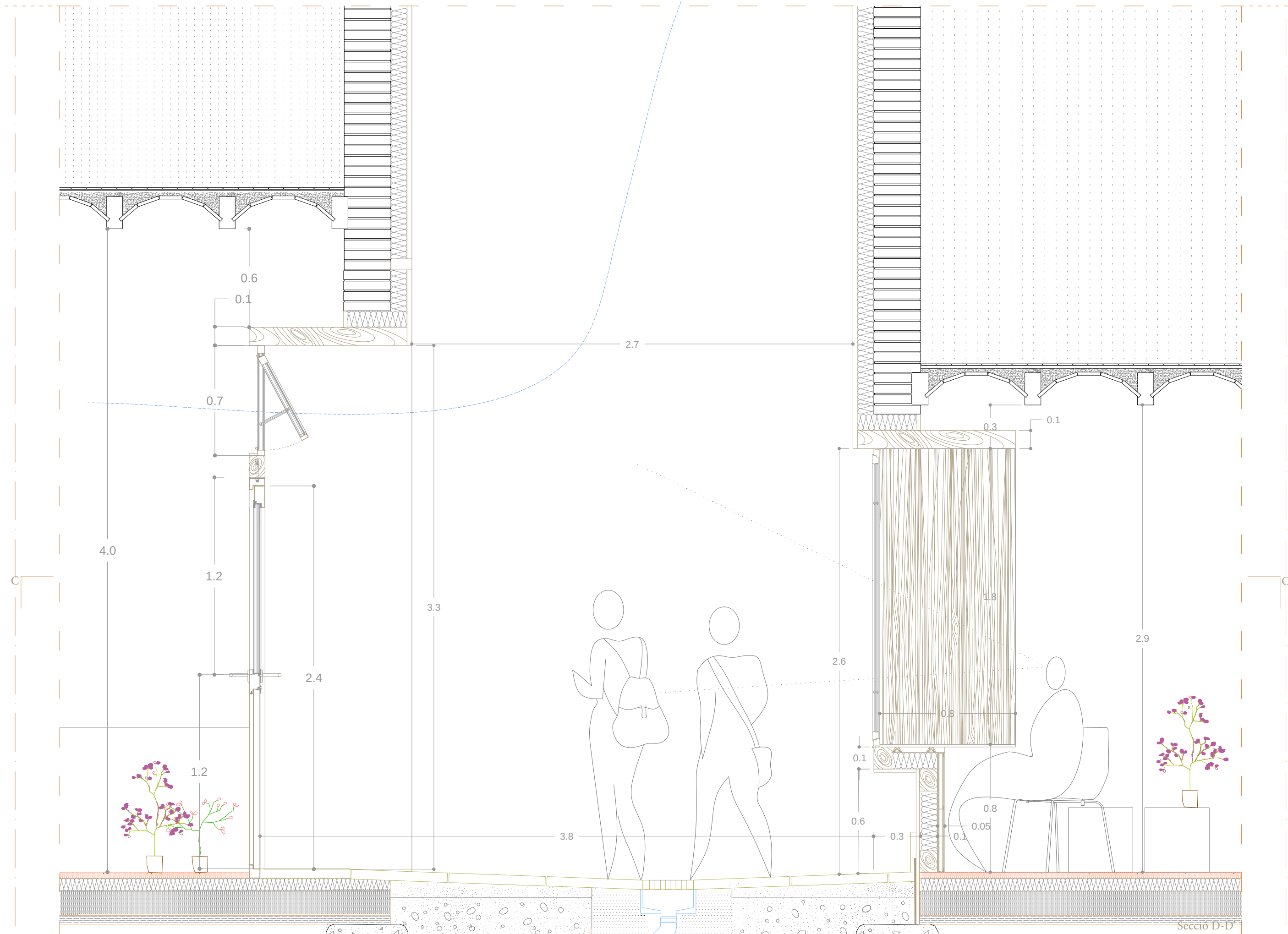
Secció D-D'
