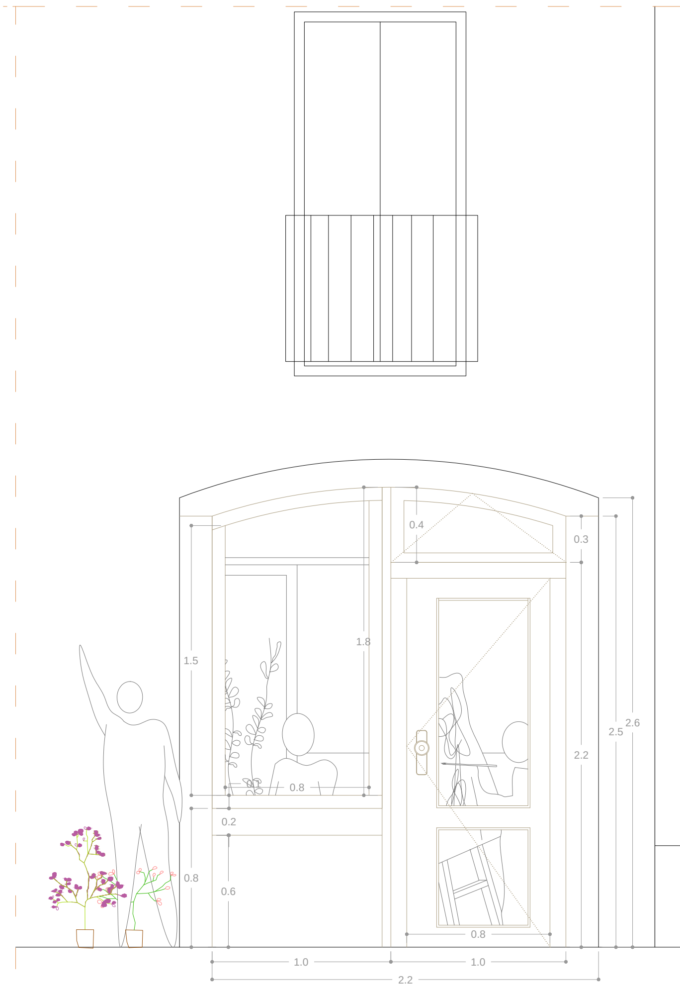
Alçat B-B'
