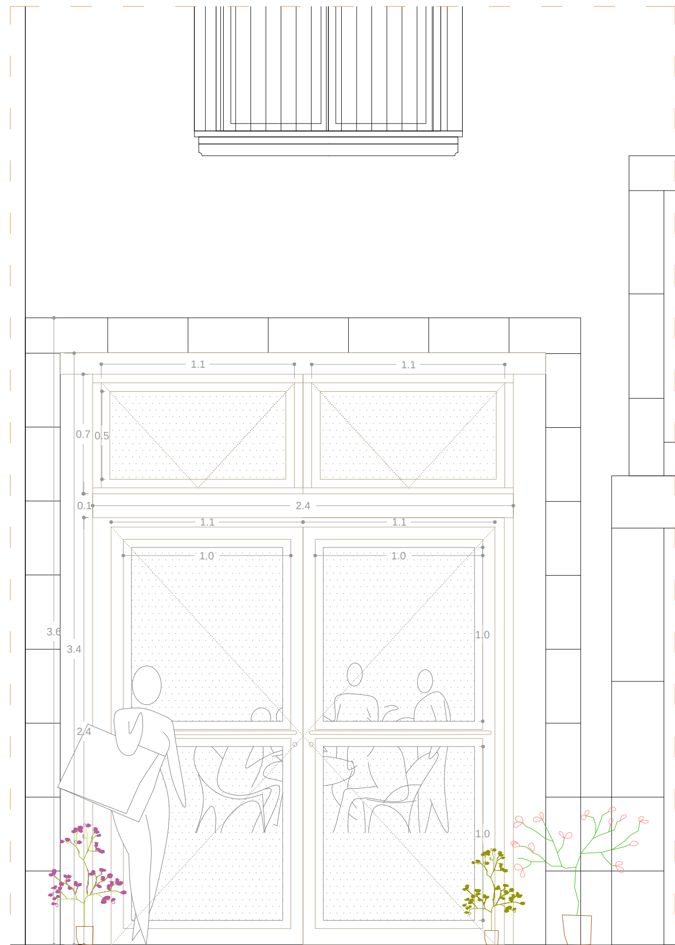
Alçat A-A'
